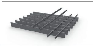
Pressroste Einfassung: T-Profil Maschenweite 20 x 20 mm Ausführung: Stahl roh und feuerverzinkt
