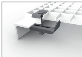
Standard-Befestigung für Maschenweite 30 x 30 mm bestehend aus: • Bügeloberteil • Sechskantschraube M8 • Vierkantmutter • Klemmunterteil
