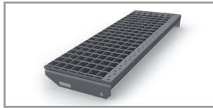
Schweißpress-Stufen Maschenweite: 30 x 30 mm mit Laschen und Antrittskante Ausführung: Stahl roh oder feuerverzinkt
