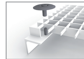
Setzbolzen-Befestigung für Maschenweite 30 x 30 mm bestehend aus: • Telleroberteil mit Gewindehülse • Gewindebolzen M8
