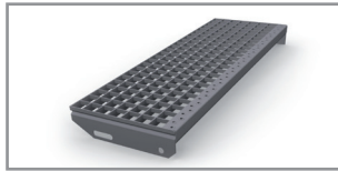
Press-Stufen Maschenweite: 30 x 30 mm mit Laschen und Antrittskante Ausführung: Stahl roh oder feuerverzinkt
