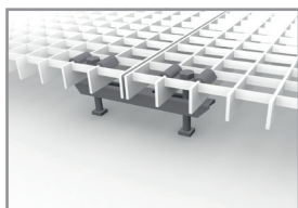
Doppelklemmen-Befestigung zur Vermeidung von Stolperkanten bei Roststößen bestehend aus: • 2 Bügeloberteilen • 2 Sechskantschrauben • 2 Vierkantmuttern • 1 Klemmunterteil
