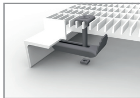
Standard-Befestigung für Maschenweite 30 x 10 mm bestehend aus: • U-Oberteil • Vierkantmutter • Klemmunterteil
