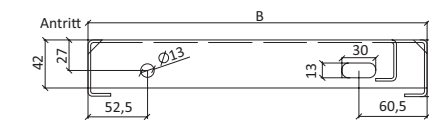
Bohrbild 2
