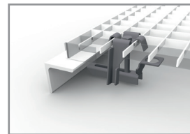
Sicherheits-Befestigung für Maschenweite 30 x 30 mm bestehend aus: • arretierendem Bügeloberteil • Sechskantschraube M8 • Vierkantmutter • Klemmunterteil
